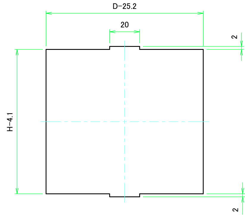
Dパネル1表面 / D Panel 1 Frontside
