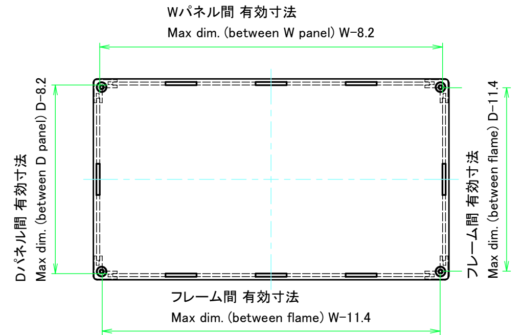
下カバー / Bottom cover
